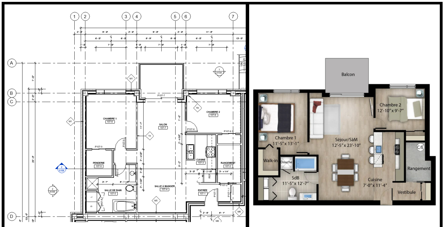
PLAN D'ÉXÉCUTION / CONSTRUCTION DRAWING
